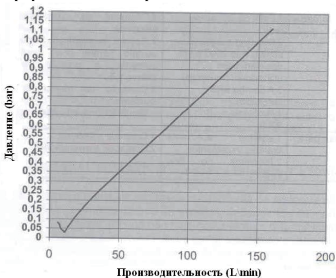
График зависимости производительности от давления
